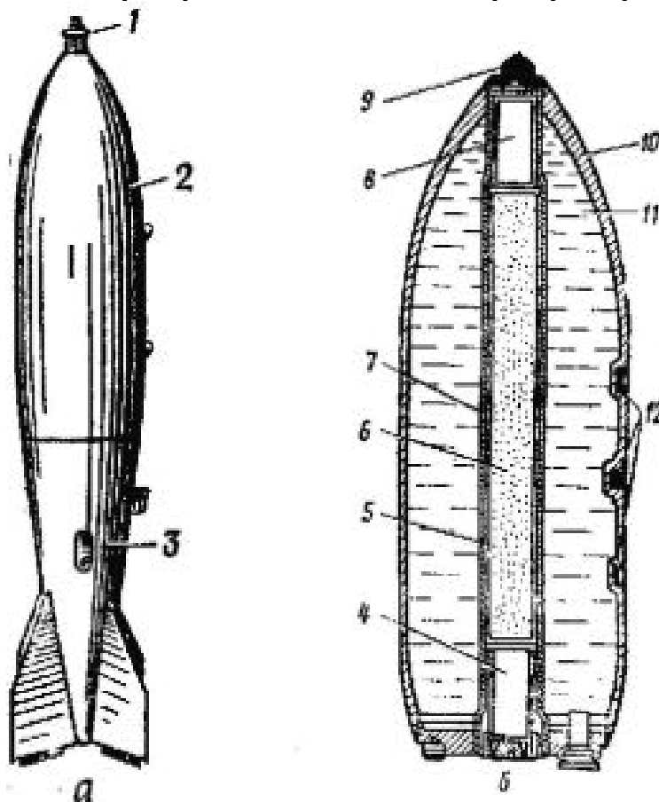
750-фунтовая химическая бомба: а) общий вид; б) устройство; 1 и 9 – взрывчатый агрегат; 2 и 10 – корпус; 3 – взрыватель; 4 и 8 – крышки для дождя и дождя в траектории; 5 – цилиндр из фибрового материала; 6 – разрывной гермет; 7 – стержень для разрывного гермет; 11 – СВ; 12 – ленточка для подвешивания
