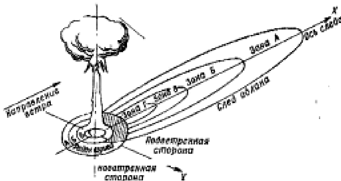
Схема радиоактивного заражения местности в районе взрыва и по следу дождя в облаке
